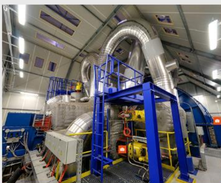
PAROPLYNOVÁ ELEKTRÁRNA POČERADY
